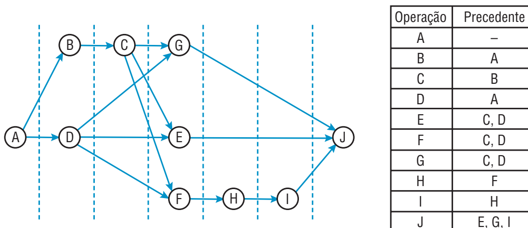
FIGURA 2 – Exemplo de um diagrama de precedência.
